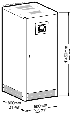
SitePro 60 kVA
