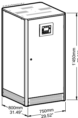
SitePro 60 kVA
